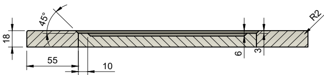
A-A (1:2)
