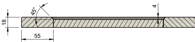
A-A (1:2)
