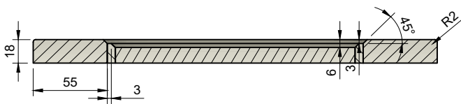
A-A (1:2)
