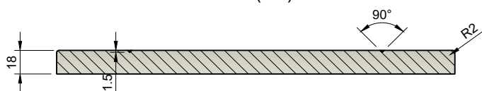
A-A (1:2)
