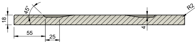
A-A (1:2)
