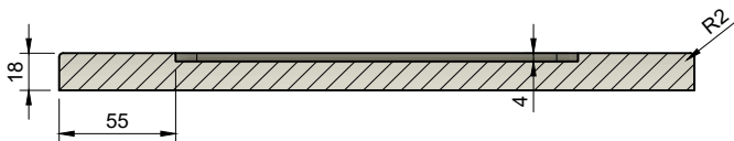
A-A (1:2)
