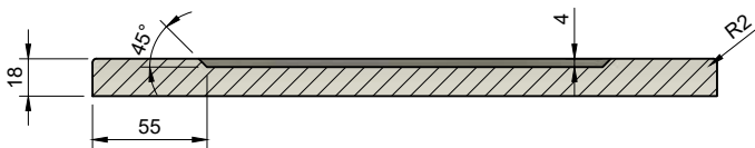
A-A (1:2)
