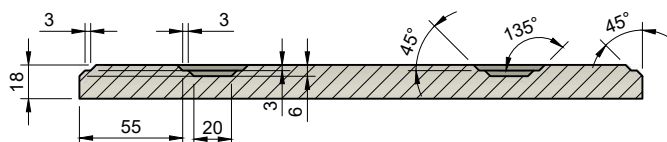
A-A (1:2)
