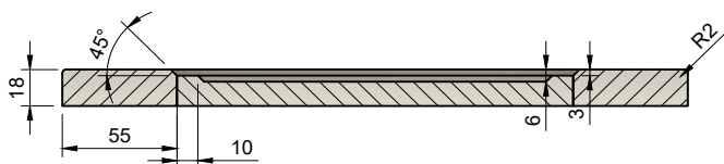
A-A (1:2)
