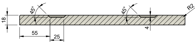
A-A (1:2)
